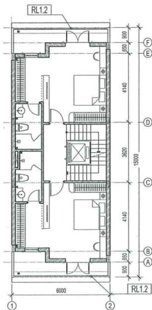
MB ĐỊNH VỊ LAN CAN TẦNG 3 TL 1/150
