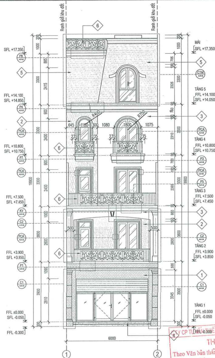
MẶT ĐỨNG TRỰC 1-2
