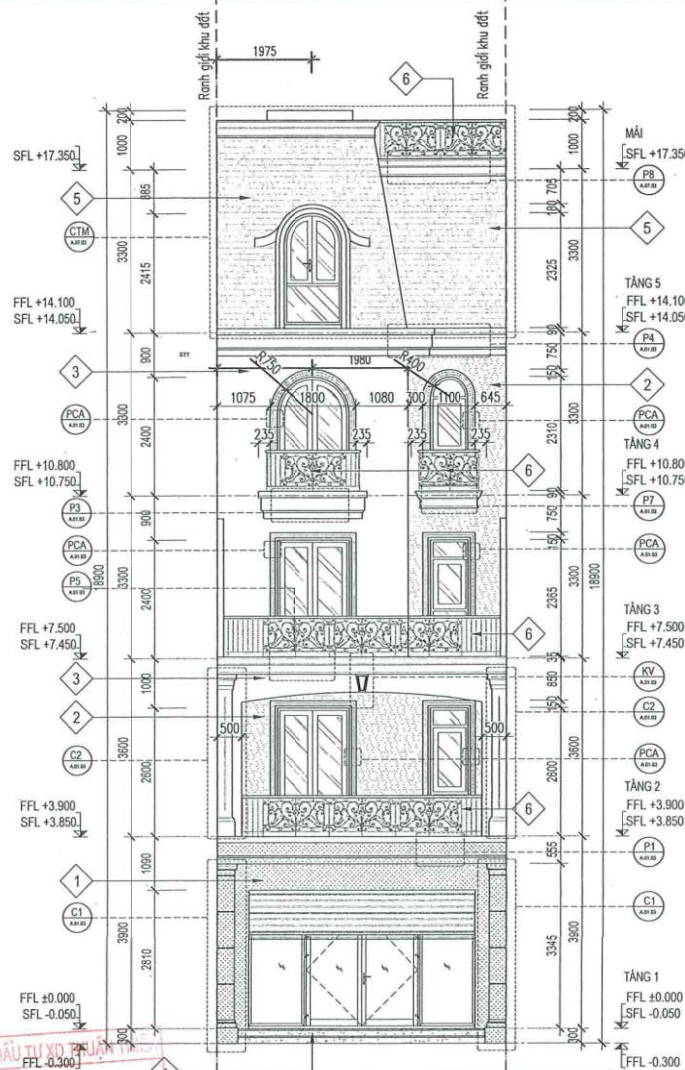
MẶT ĐỨNG TRỰC 2-1
