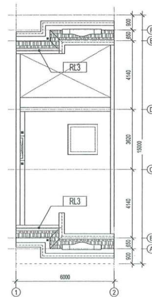
MB ĐỊNH VỊ LAN CAN MÁI TL 1/150
