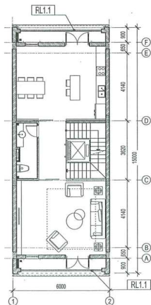
MB ĐỊNH VỊ LAN CAN TẦNG 2 TL 1/150
