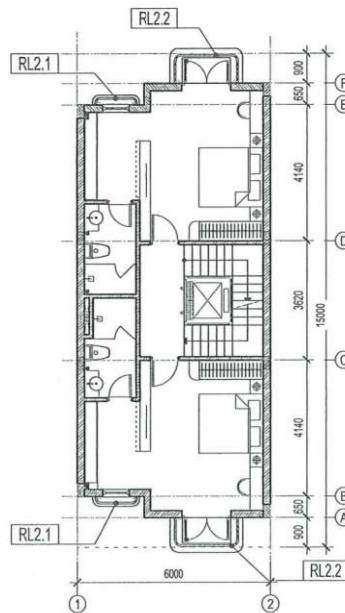
MB ĐỊNH VỊ LAN CAN TẦNG 4 TL 1/150
