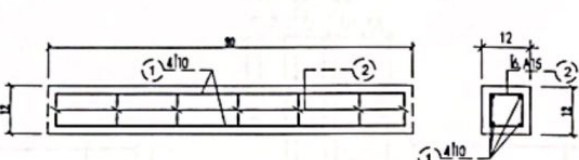
THÔNG KÊ CỐT THÉP THANH GIẢNG (TÍNH CHO 10M KÈNH)
