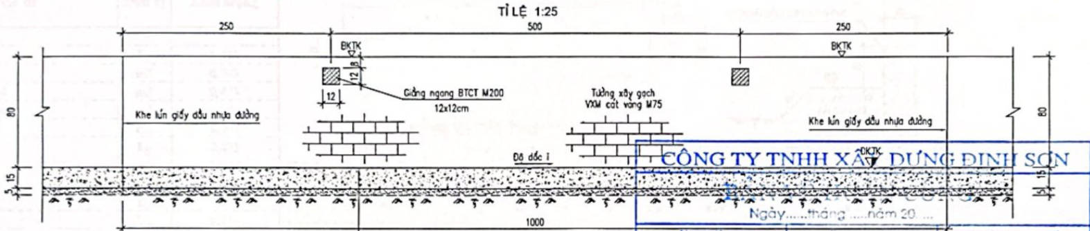
CẮT DỌC ĐIỂN HÌNH KÈNH CNXG 06
