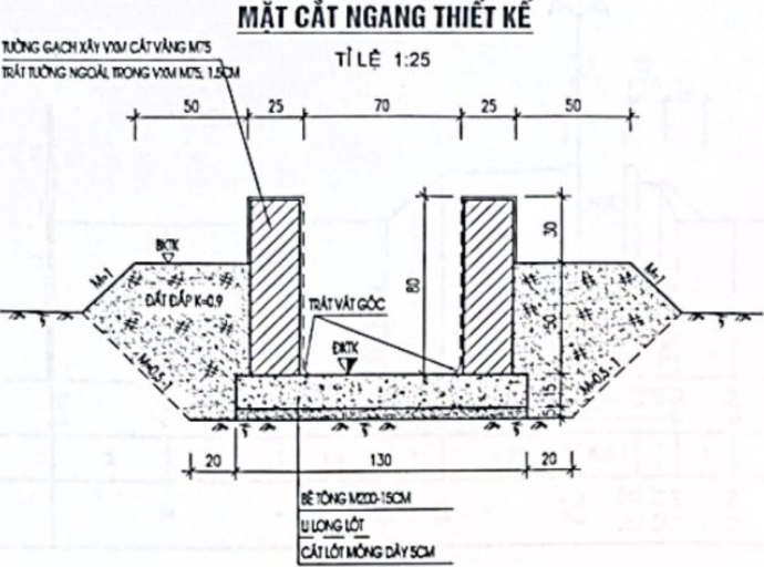
CHI TIẾT GIẢNG
