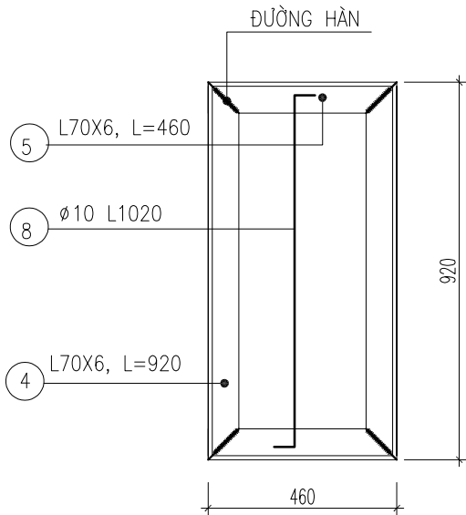
KHUNG THÉP VIÊN
