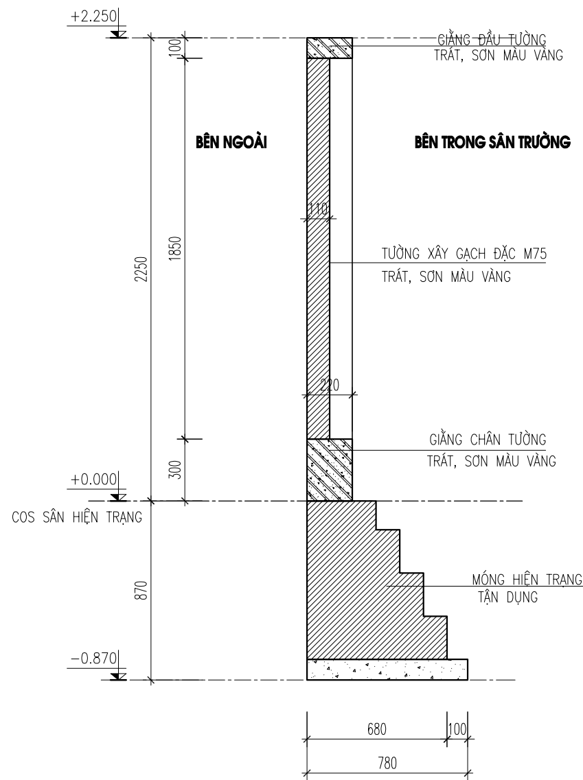
CHI TIẾT TƯỜNG RÀO ĐẶC CHIỀU DÀI, L= 84M
