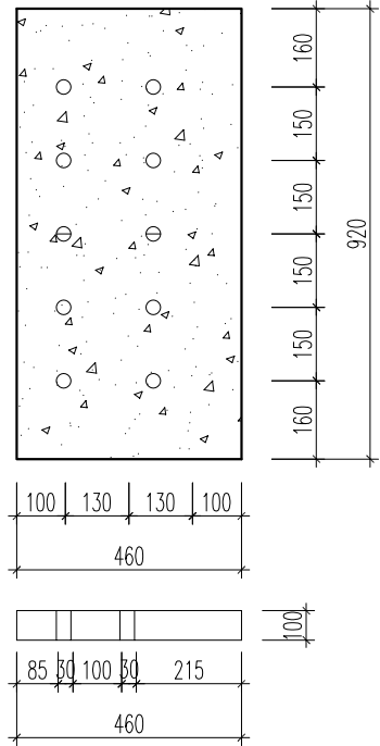
CẤU TẠO TẮM ĐAN
