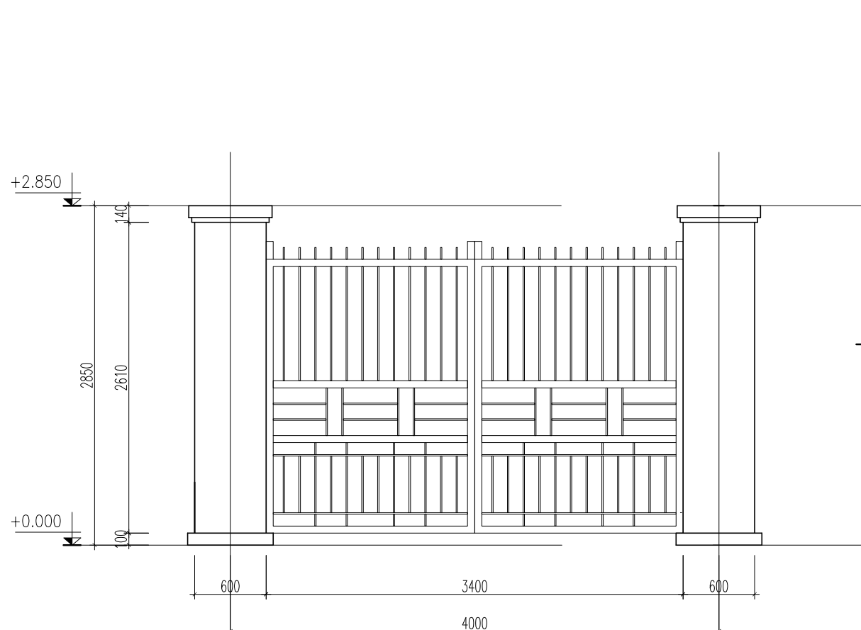
MẶT ĐỨNG CỔNG
