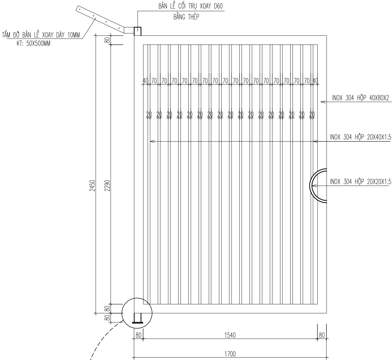
CÁNH CỔNG, SL: 2CK
