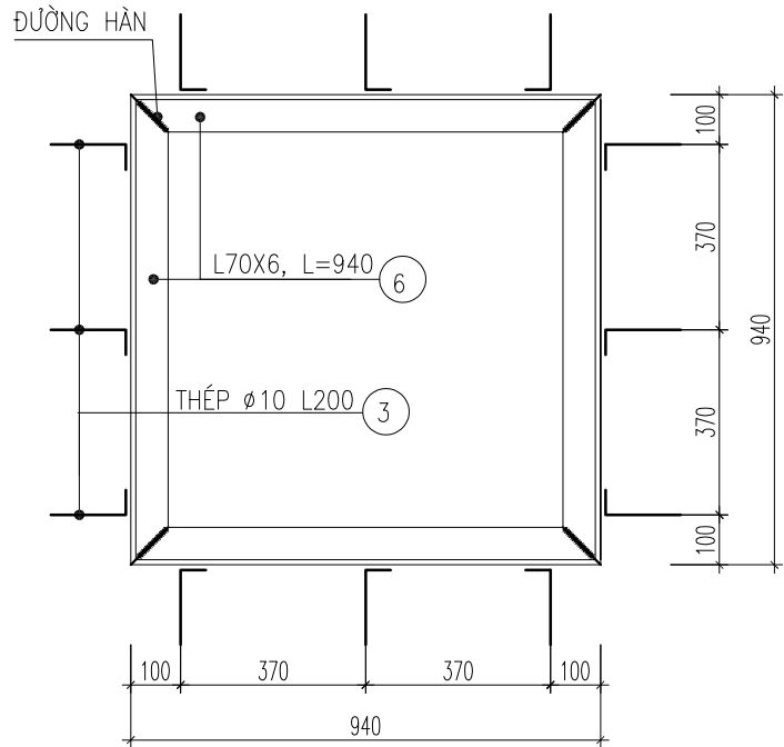
KHUNG THÉP VIÊN MIỆNG GA
