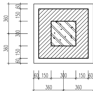
MC A-A
