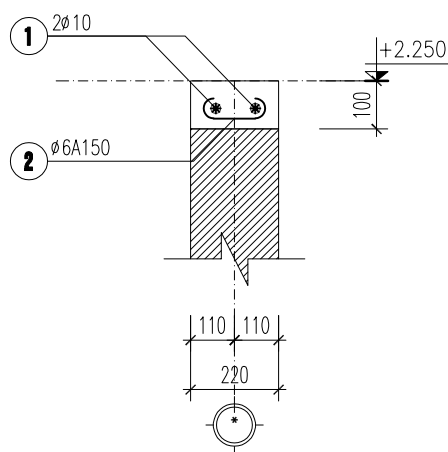
CHI TIẾT GIĂNG ĐẦU TƯỜNG GT
