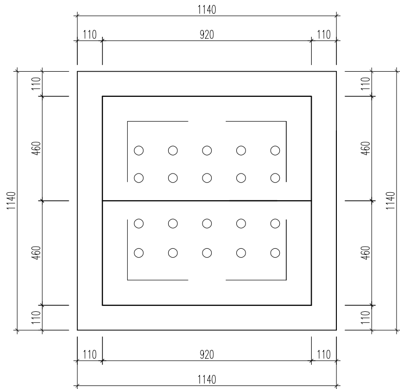
MB BỐ TRÍ TẮM ĐAN GA 01
