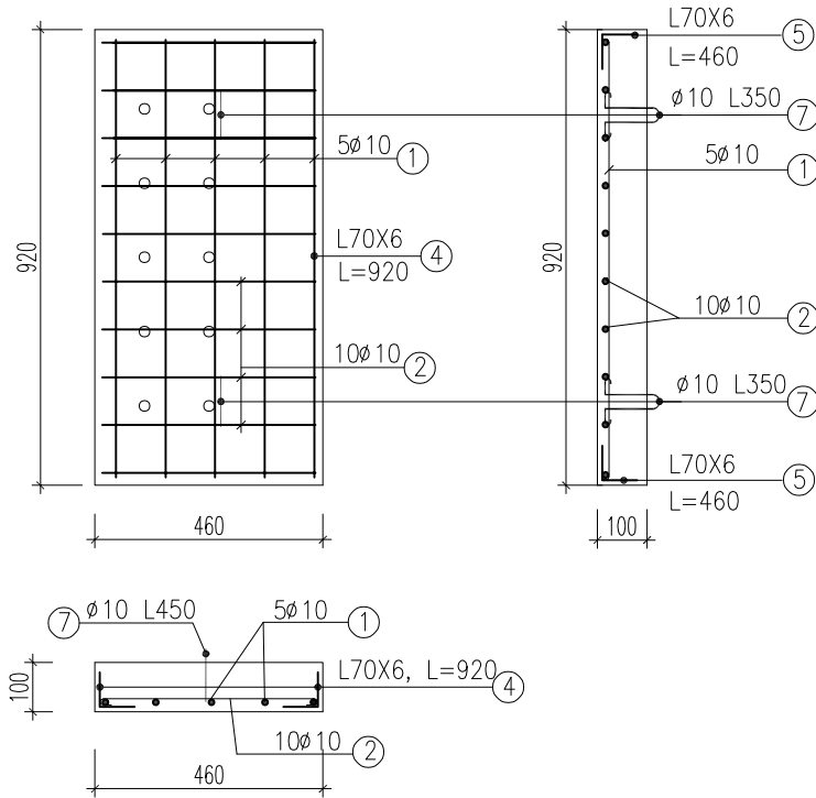
CT CỐT THÉP TẮM ĐAN
