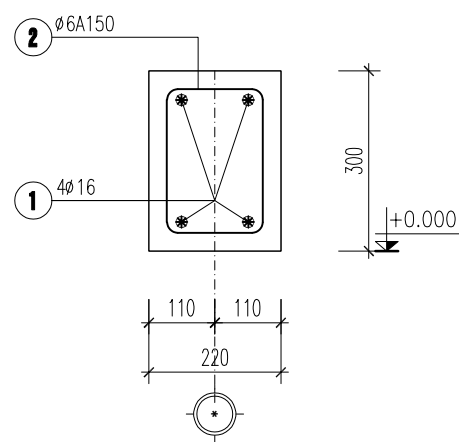
CHI TIẾT GIĂNG CHÂN TƯỜNG GM
