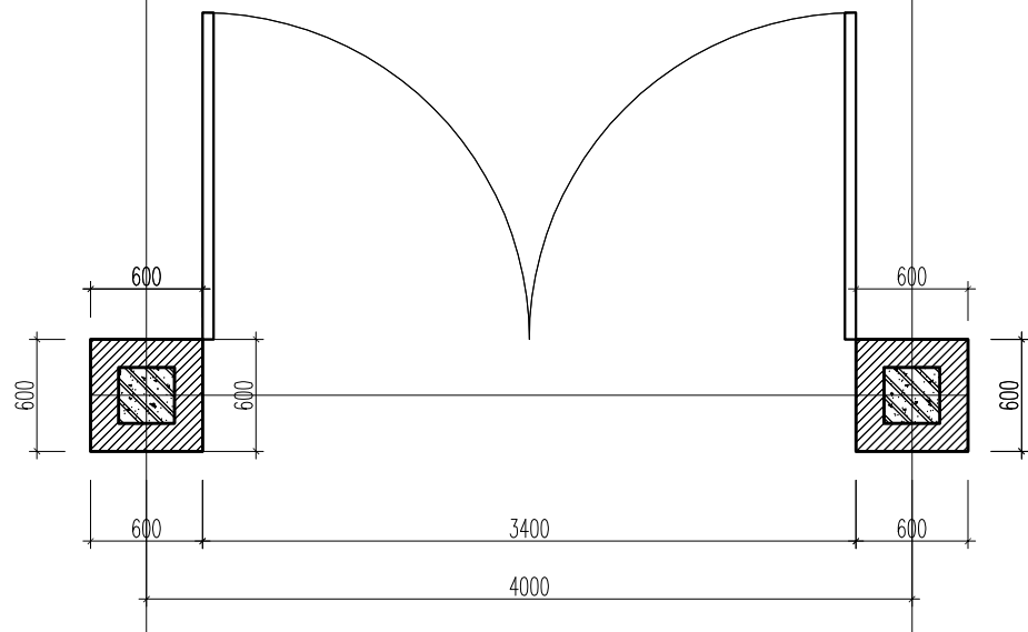
MẶT BẰNG CỔNG
