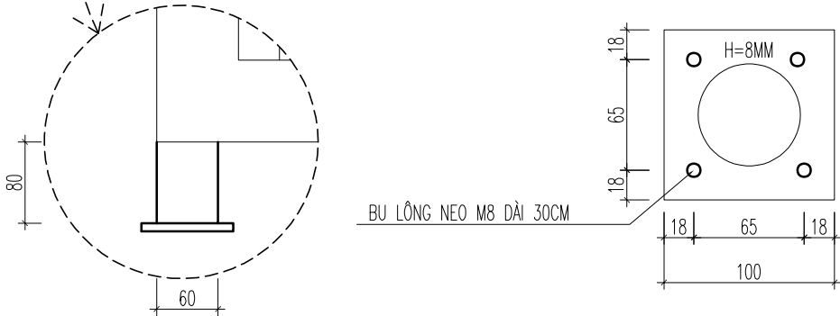
CHI TIẾT BẢN MÃ
