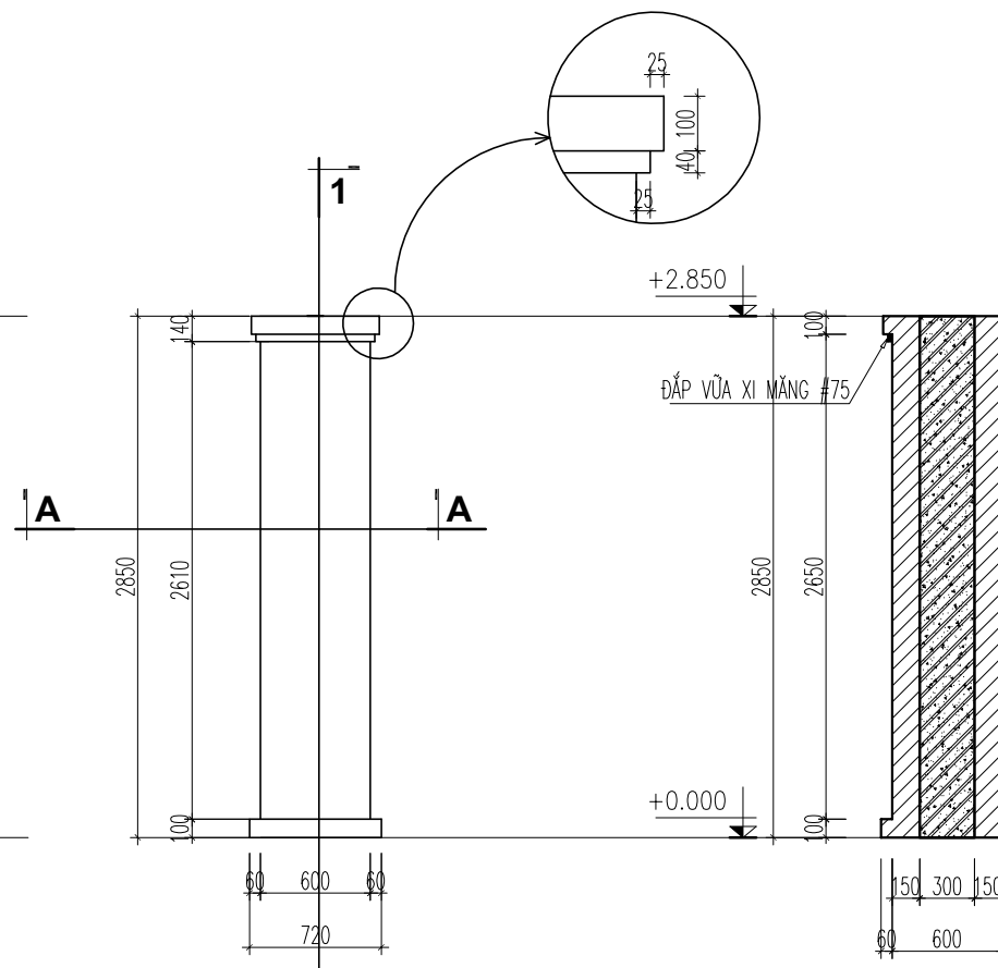
CT TRỤ CỔNG
